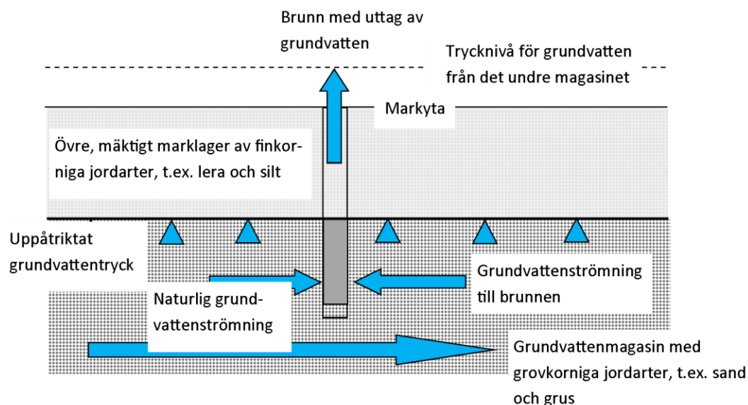
Figur 8: Schematisk bild över hur grundvattenbalansen är uppbyggd för en artesisisk grundvattentäkt.
